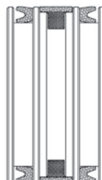
Piston
