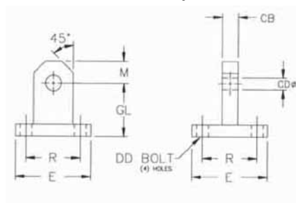
Detachable Eye
