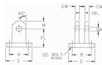
Detachable Clevis
