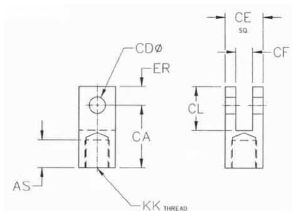
Rod Clevis
